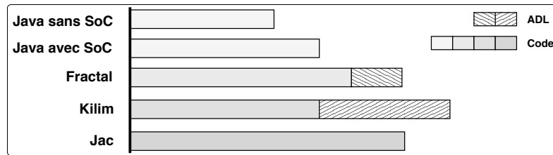
Figure 2. Quantité de lignes de code en fonction de la plate-forme d'accueil.
